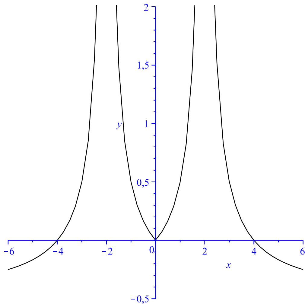
Grafico di f(x) = \frac{1}{||x| - 2|} - \frac{1}{2}
