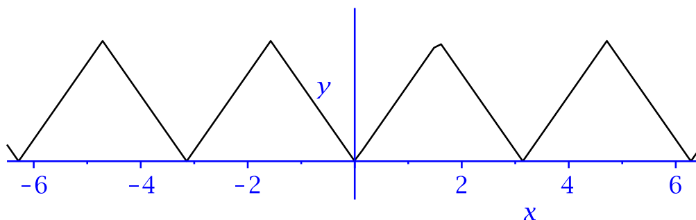
Grafico di f(x) = \arctan(|\tan(x)|)
